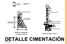
DETALLE CIMENTACIÓN
