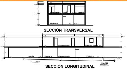
SECCIÓN LONGITUDINAL
